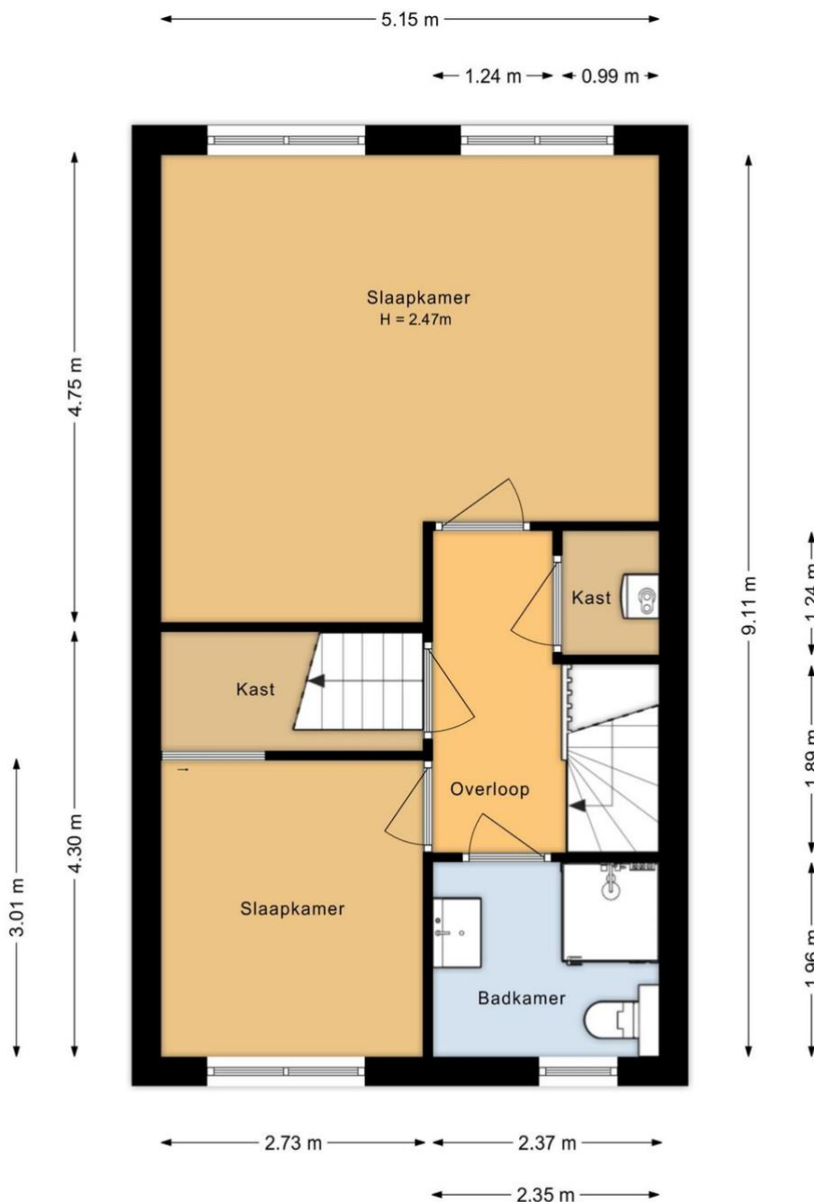
Eerste verdieping Paviljoentjalk 2 Velserbroek
